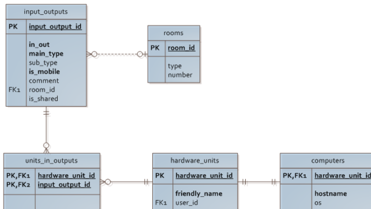
FIG. 4.15 – Le schéma infrastructure de la base de données – partie « matériel ».
