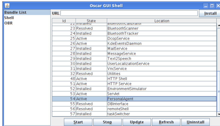
FIG. 4.12 – Interface graphique de visualisation et manipulation des bundles OSGi.
