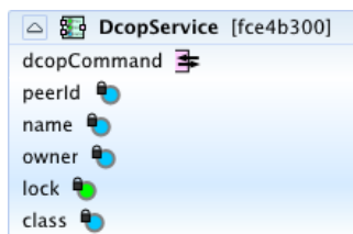
FIG. B.10 – Le service DcopService dans OMISCIDGui.
