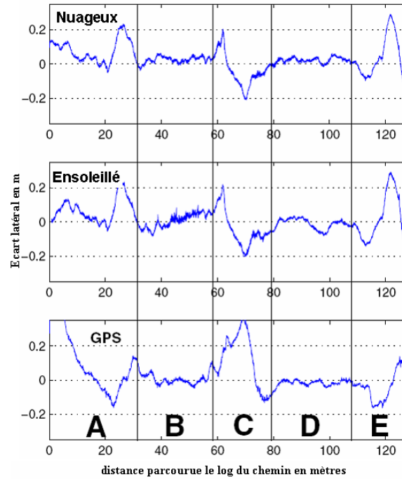
FIG. 4.24 – Ecarts latéraux avec le chemin référence
