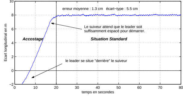
FIG. 4.31 – Ecart longitudinal
