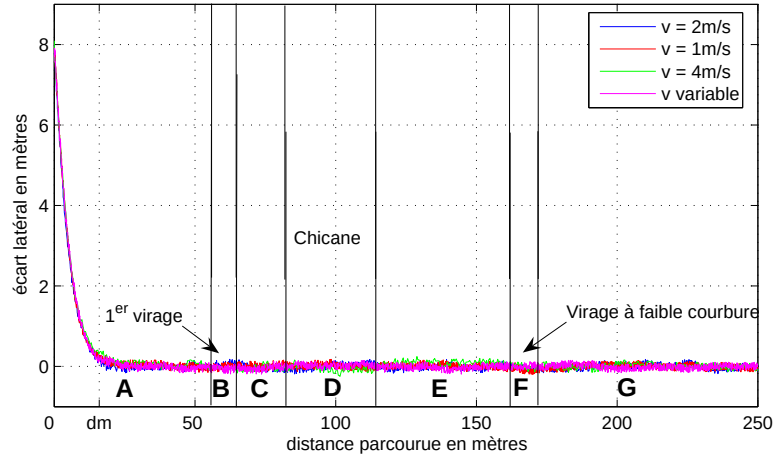
FIG. 2.16 – Erreur latérale en fonction de la distance parcourue - Simulation 3
