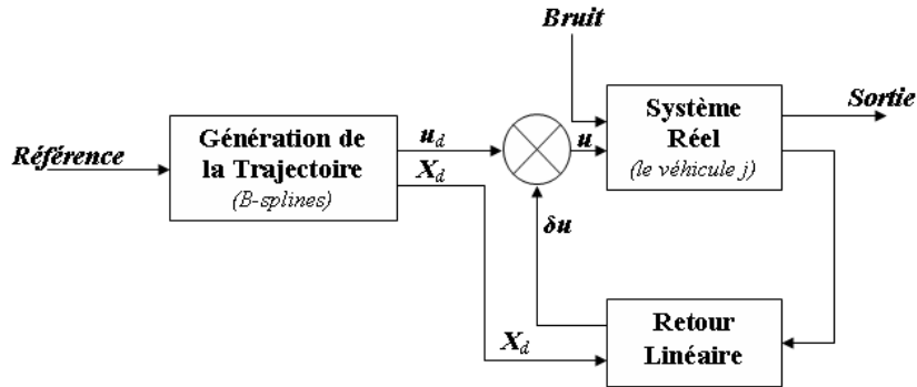
FIG. 1.21 – Schéma de commande par platitude
