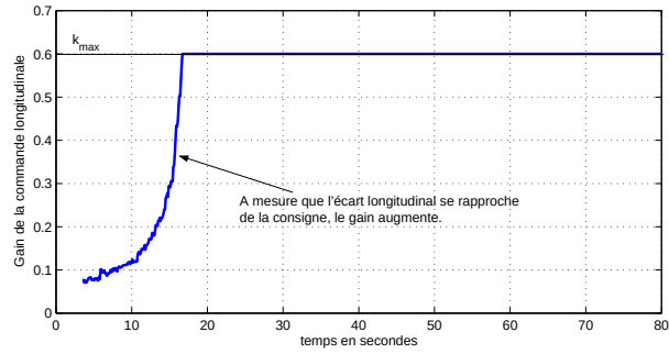
FIG. 4.32 – Gain adaptatif
