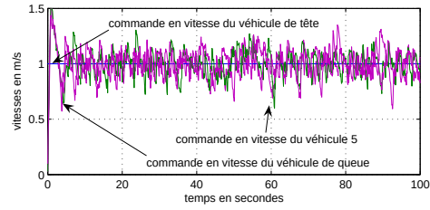
FIG. 2.30 – Commandes en vitesse appliquées - Simulation 6
