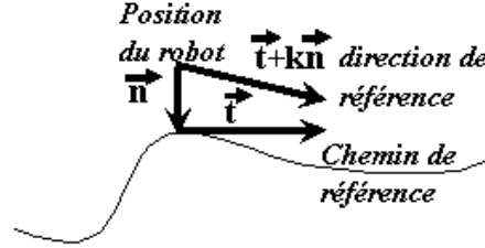
FIG. 1.18 – Détermination de l'orientation de référence
