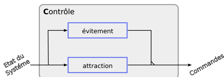
FIGURE 1.11 – Architecture subsumption pour le déplacement d'un robot mobile dans un environnement encombré
