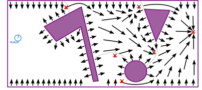
FIGURE 1.19 – Champ de force après propagation dans la seconde zone
