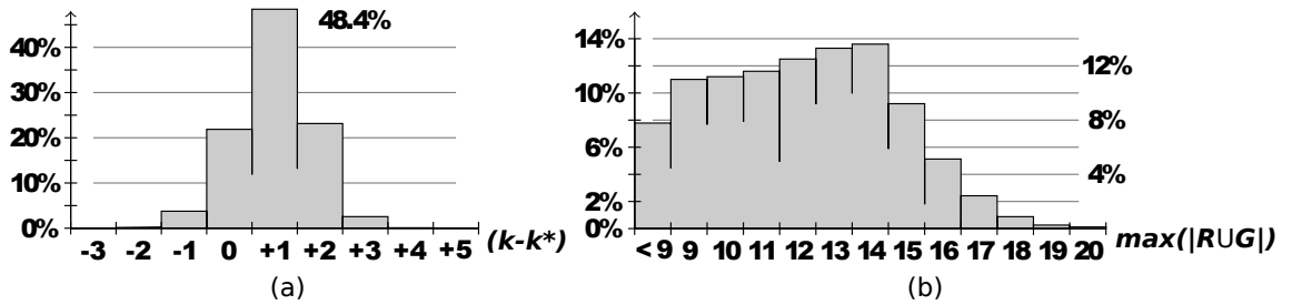
FIGURE 4.9 – Tailles des partitions gloutonnes créée. Les diagrammes (a) et (b) classifient les expériences en fonction : (a) de la différence entre le nombre construit k et le nombre idéal k^* de régions et (b) le nombre d'objectifs contenus dans la région la plus importante. Par exemple, (a) 48.4% des partitionnements ont construit une région de trop par rapport au nombre idéal k^* et (b) 13.5% des régions possèdent 14 objectifs.
