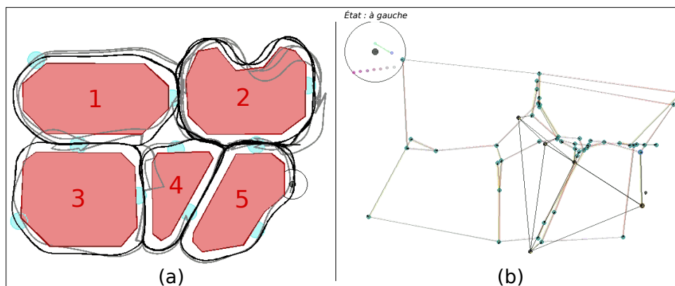
FIGURE 3.29 – Exploration dans un état avancé. Due à l’orientation des nœuds dans la Road-Map , le robot doit explorer les chemins topologiques dans les 2 directions possibles. À cette étape de la mission, tous les obstacles ont été encadrés mais il reste des positions frontières dans les orientations opposées. En effet, encadré un obstacle dans un sens (par la gauche par exemple) ne permet pas actuellement, de définir les nœuds et connexions dans le sens opposé. Ici, seul l’obstacle 2 a été encadré dans les deux directions et le robot continue son exploration.
