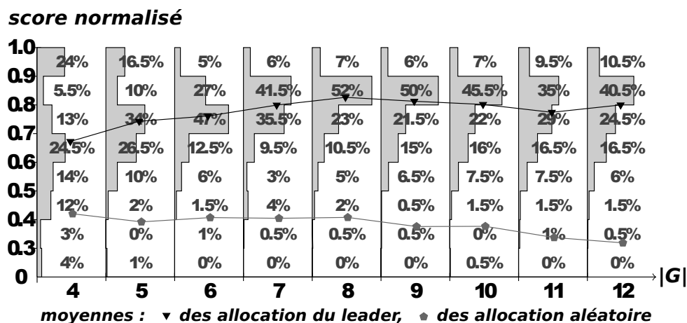
FIGURE 4.8 – Évaluation des allocations résultant d'un partitionnement glouton. La population des scores obtenus par une allocation basée sur un GO-MDP abstrait approché est présentée en fonction du nombre d'objectifs considérés |G| . Par exemple pour |G| = 8 : 7% des allocations construites ont eu un score entre 0.9 et 1.0 (avec 1.0 : allocation optimale) ; 52% entre 0.8 et 0.9, etc.
