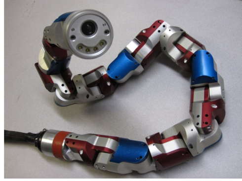
FIGURE 1.6 – Uncle Sam : robot biomorphe hyper-redondant ressemblant à un serpent développé par Biorobotics Laboratory, Carnegie Mellon University
