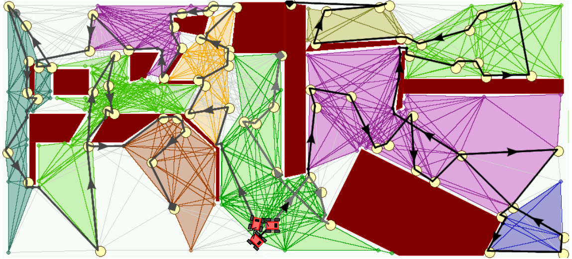
FIGURE 4.6 – Résolution hiérarchique, exemple de parcours empruntés par les 3 robots après répartition des régions par le leader et calcul individuel des politiques locales.
