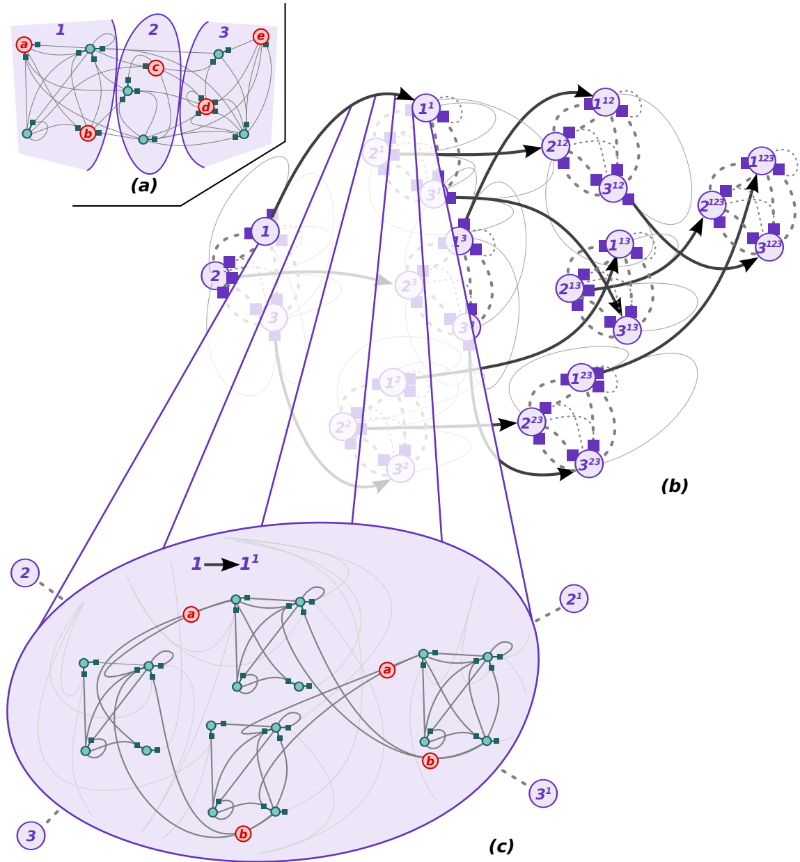
FIGURE 4.4 – Combinaison du GO-MDP abstrait (b) et d'un GO-MDP local (c) correspondant à l'état abstrait (1, \emptyset) . Ces 2 GO-MDPs dépendent des modifications réalisées sur le MDP système décomposé (a) et ses 5 objectifs G = \{a, b, c, d, e\} .
