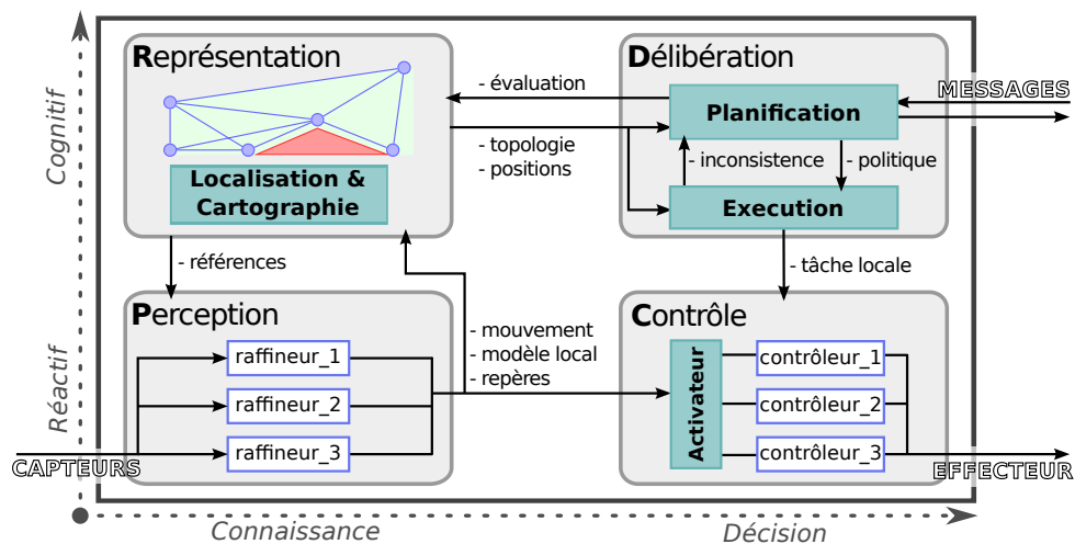
FIGURE 3.4 – Architecture PRDC "2 axes" (Connaissance/Décision \times Réactif/Cognitif).
