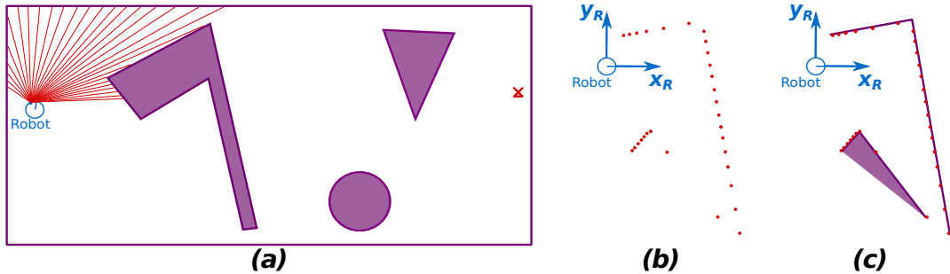
FIGURE 1.28 – (a) exemple de mesure perçus par un capteur télémétrique par rapport (b) à sa position dans l'environnement et (c) la forme géométrique des obstacles sensée être reconstituée à partir de la donnée.
