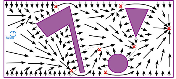
FIGURE 1.21 – Champ de force total après propagation.
