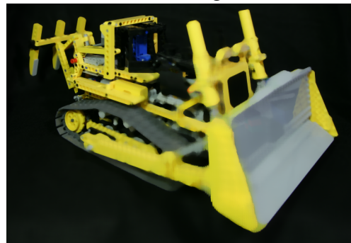
(d) Median
