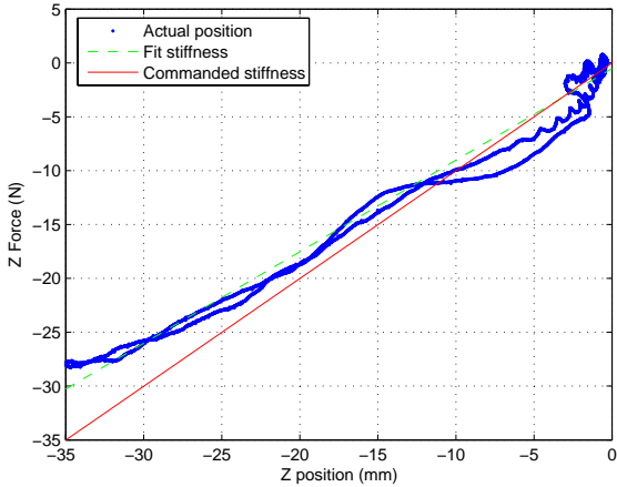
Fig. 6. Actual rendered stiffness at 1000\text{ N/m}
