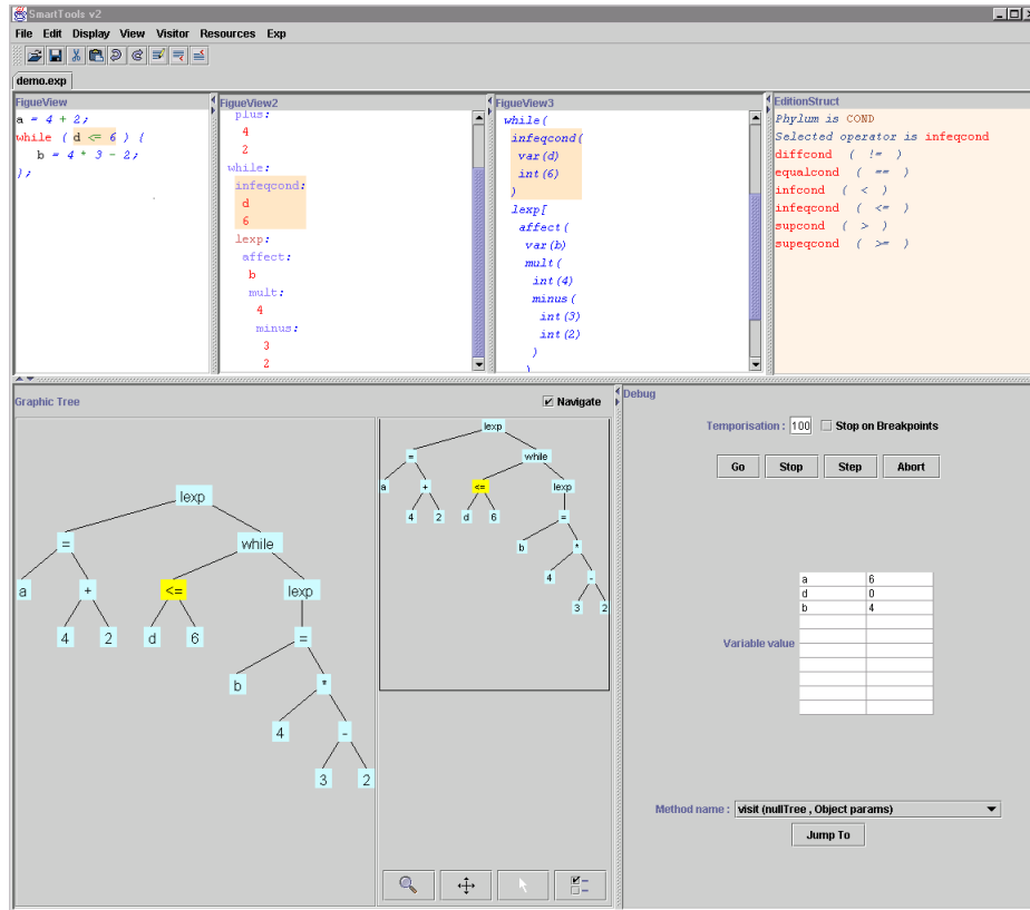
Fig. 1. SmartTools
