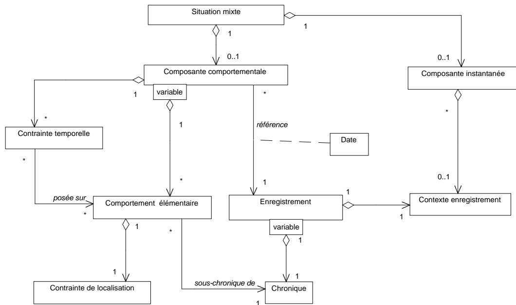
Figure 6 : diagramme des classes pour la représentation des situations comportementales
