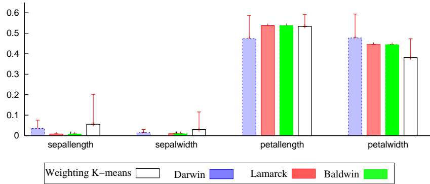
FIG. 3 – Iris : Moyenne et variance des poids trouvés sur chacun des attributs (100 expériences)
