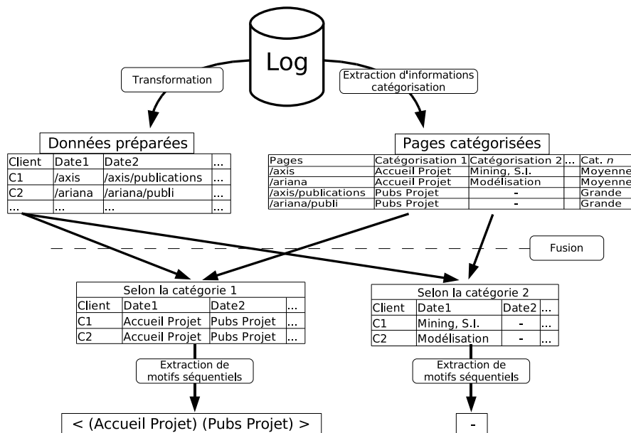
FIG. 3 – Méthodologie de catégorisation et d'analyse des usages
