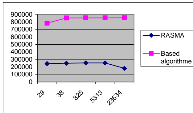
FIG. 3 – temps d'exécution en fonction de la taille cible
