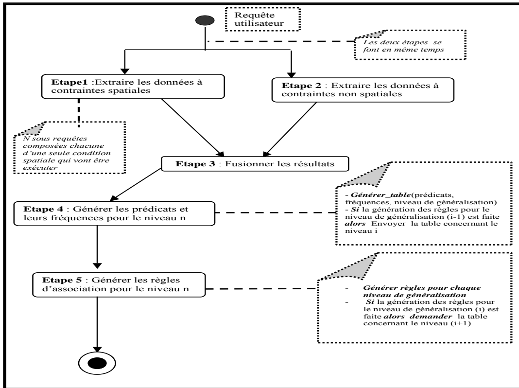
FIG. 1 – Algorithme d'extraction des règles d'association spatiales
