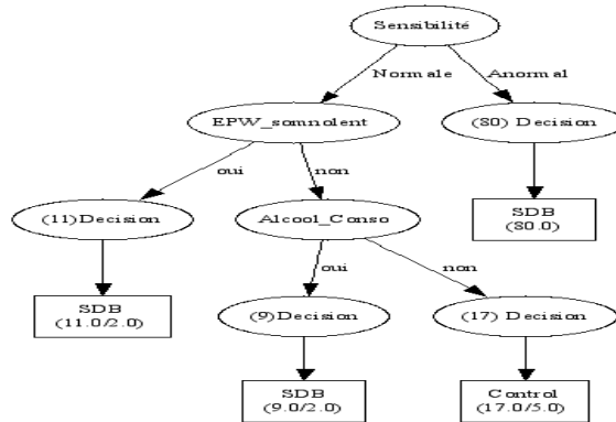
FIG. 2 – L'Arbre de Décision Probabiliste AAP (base apnées du sommeil).
