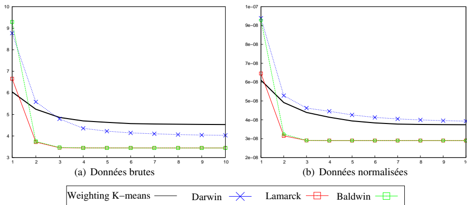
FIG. 2 – Iris : Evolution de la fonction WCost pour les différents algorithmes
