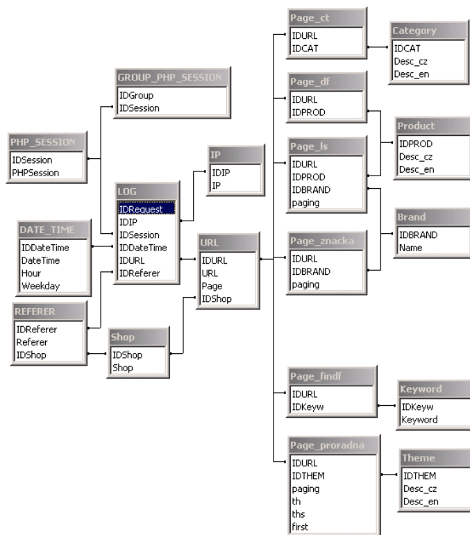
FIG. 1 – Model relationnel de la base de donnée.
