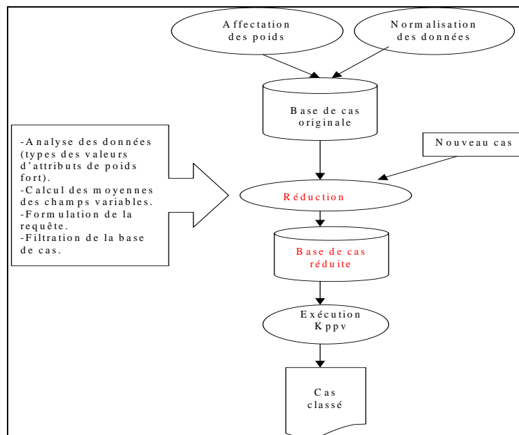
Figure 2 : processus de classification par Kppv proposé
