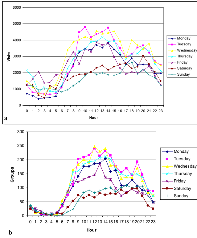
FIG. 3 – Visites par jour et heure e: (a) globalement, (b) multi-site.
