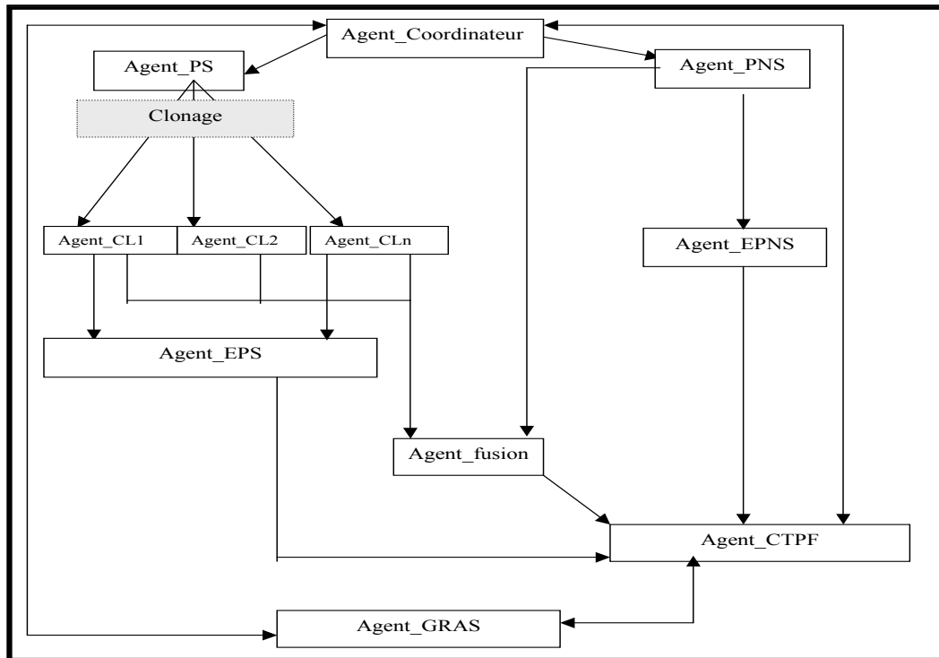
FIG. 2 – Architecture du système multi-agent RASMA
