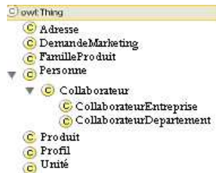
Figure 3 : Ontologie globale
