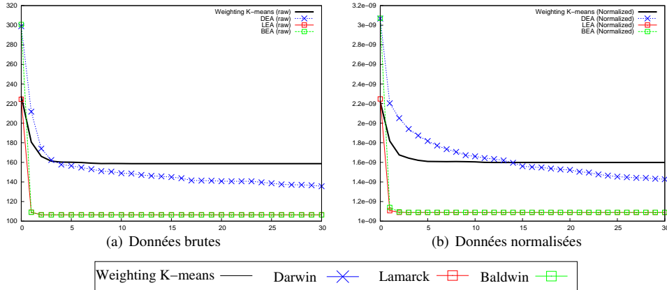
FIG. 4 – Diabetes : Evolution de la fonction WCost pour les différents algorithmes
