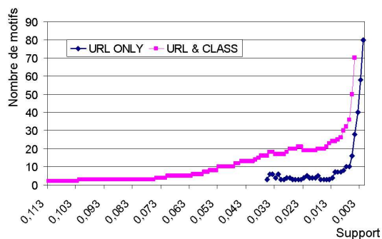
FIG. 4 – Nombre de motifs extraits à différents supports avec et sans généralisation des URLs
