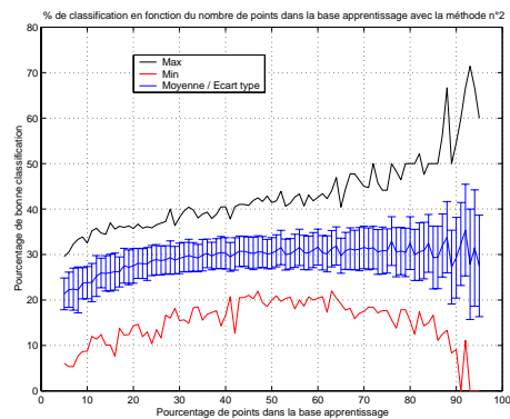
FIG. 2 – Pourcentage de bonne classification en fonction du nombre de points dans la base d'apprentissage pour la méthode n 2 .
