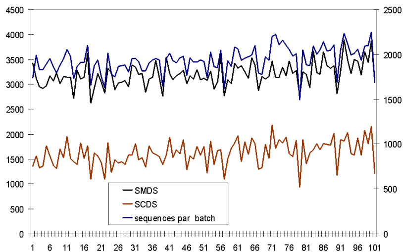
FIG. 3 – Temps d'exécution de SCDS.
