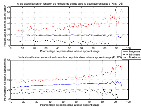
FIG. 5 – Pourcentage de bonne classification en fonction du nombre de points dans la base d'apprentissage pour les KNN-DS et ProDS.
