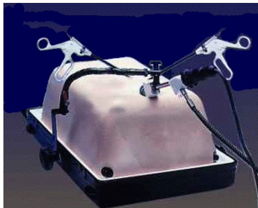
FIG. 4 – Simulateur mécanique de chirurgie laparoscopique (© 1997 United States Surgical Corporation).
