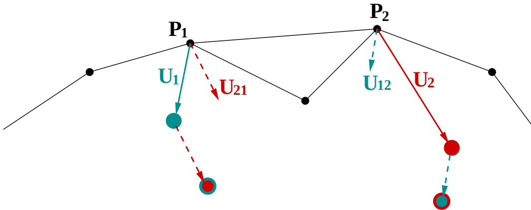
FIG. 2.5 – Problème posé par l'application de déplacements sur deux sommets simultanément
