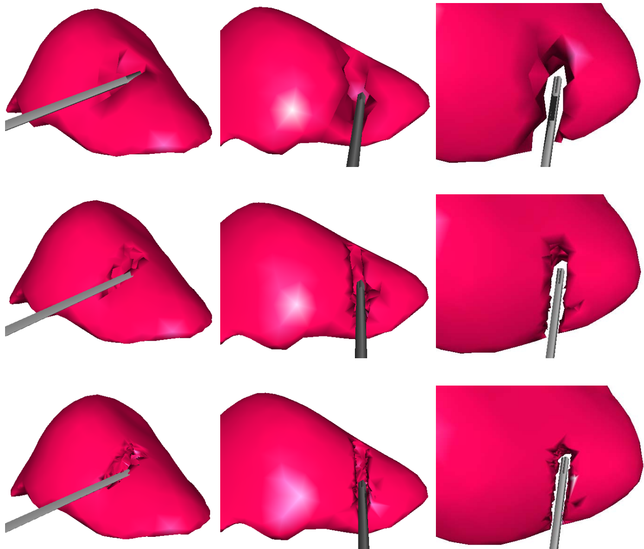
FIG. 4.14 – Exemple de découpe du foie. La première ligne montre la découpe sur le maillage de départ. Sur la deuxième et la troisième lignes la découpe est couplée avec l'algorithme de raffinement automatique de la zone en contact avec l'outil : chaque arête est subdivisée une fois pour la deuxième ligne et deux fois pour la troisième.
